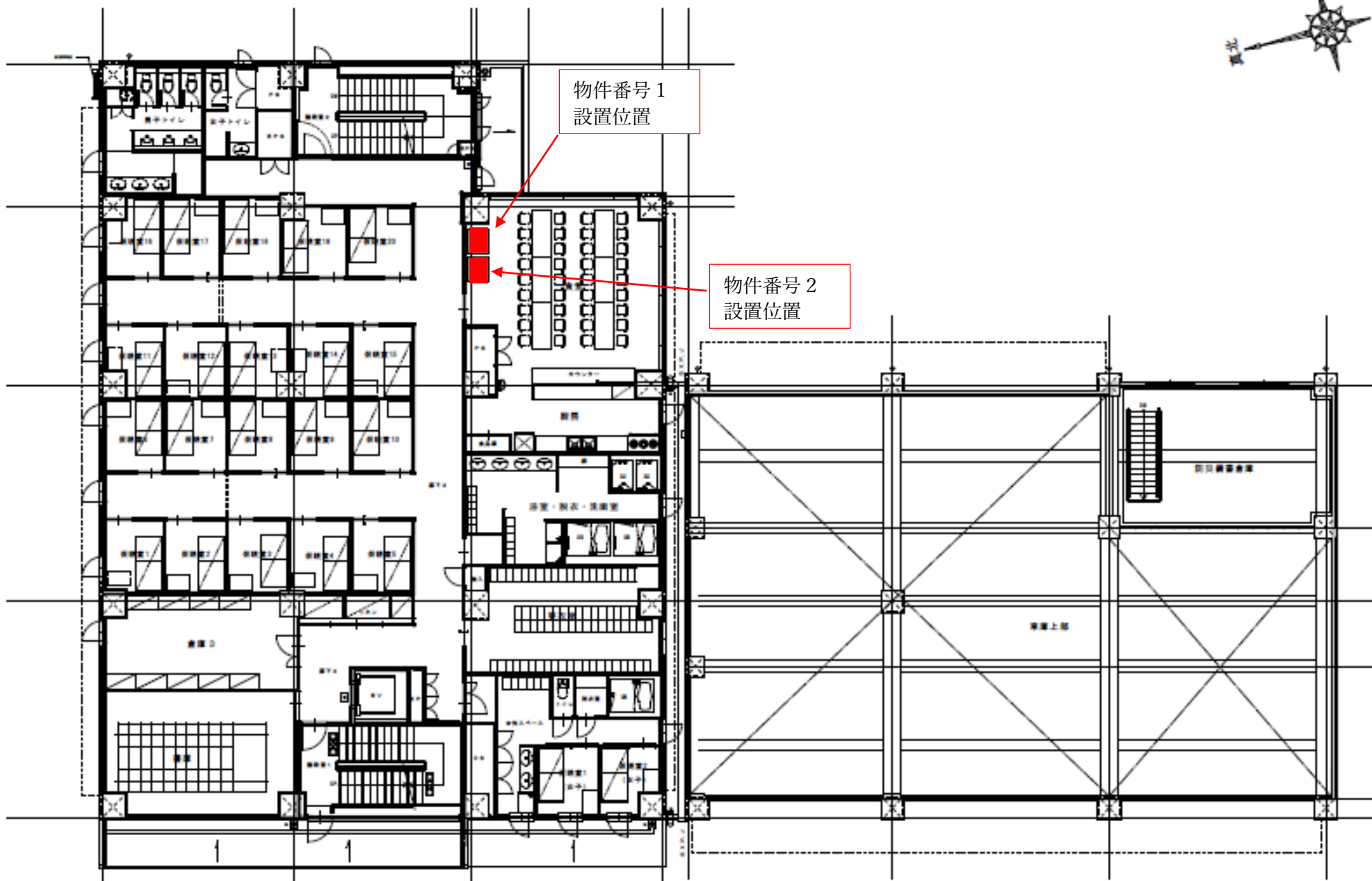
2 階 平 面 図
