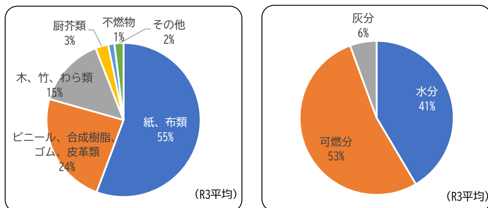
図3-2-6 事務組合におけるごみ質調査結果
