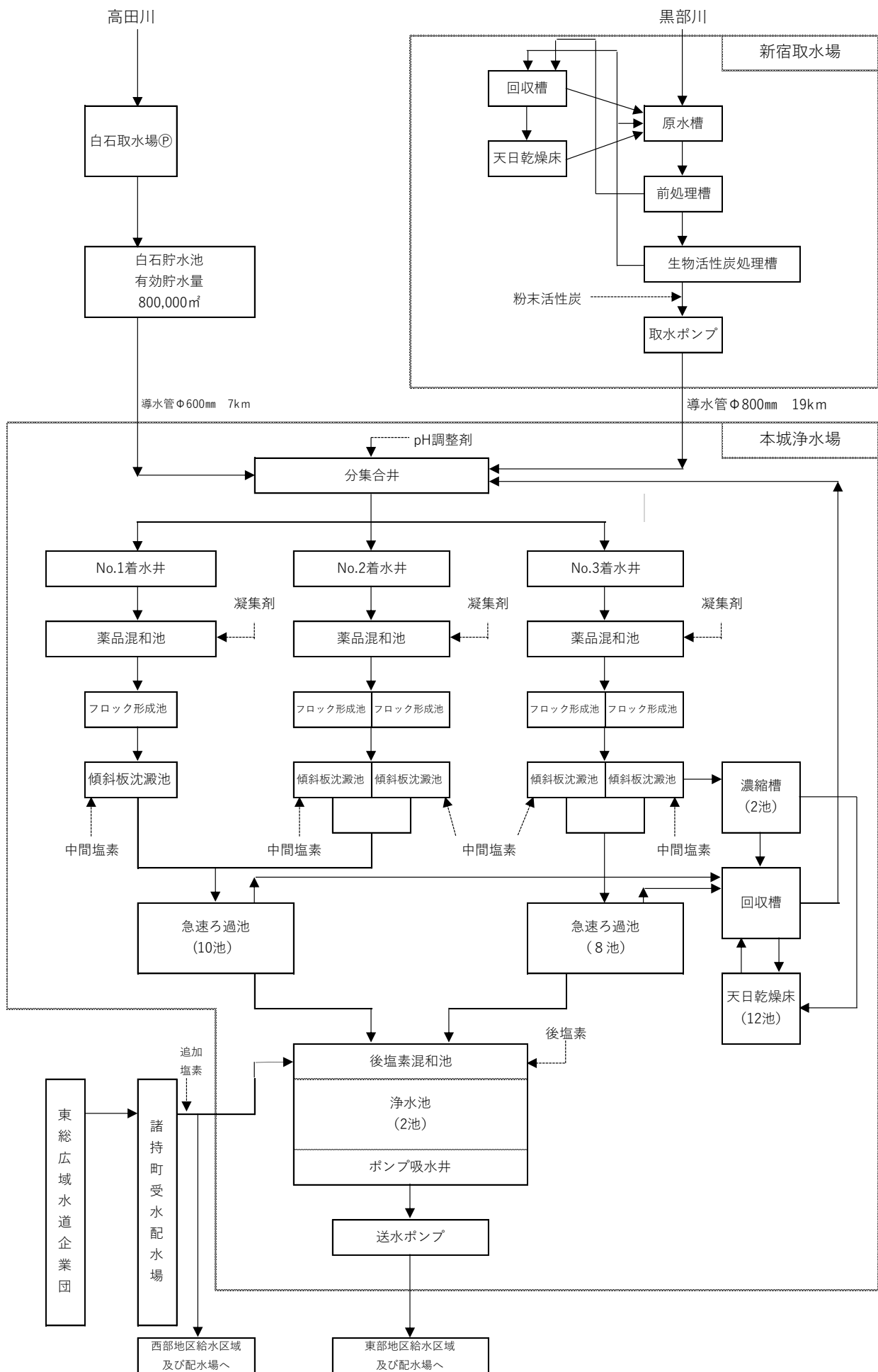
図2 浄水方法フロー図
