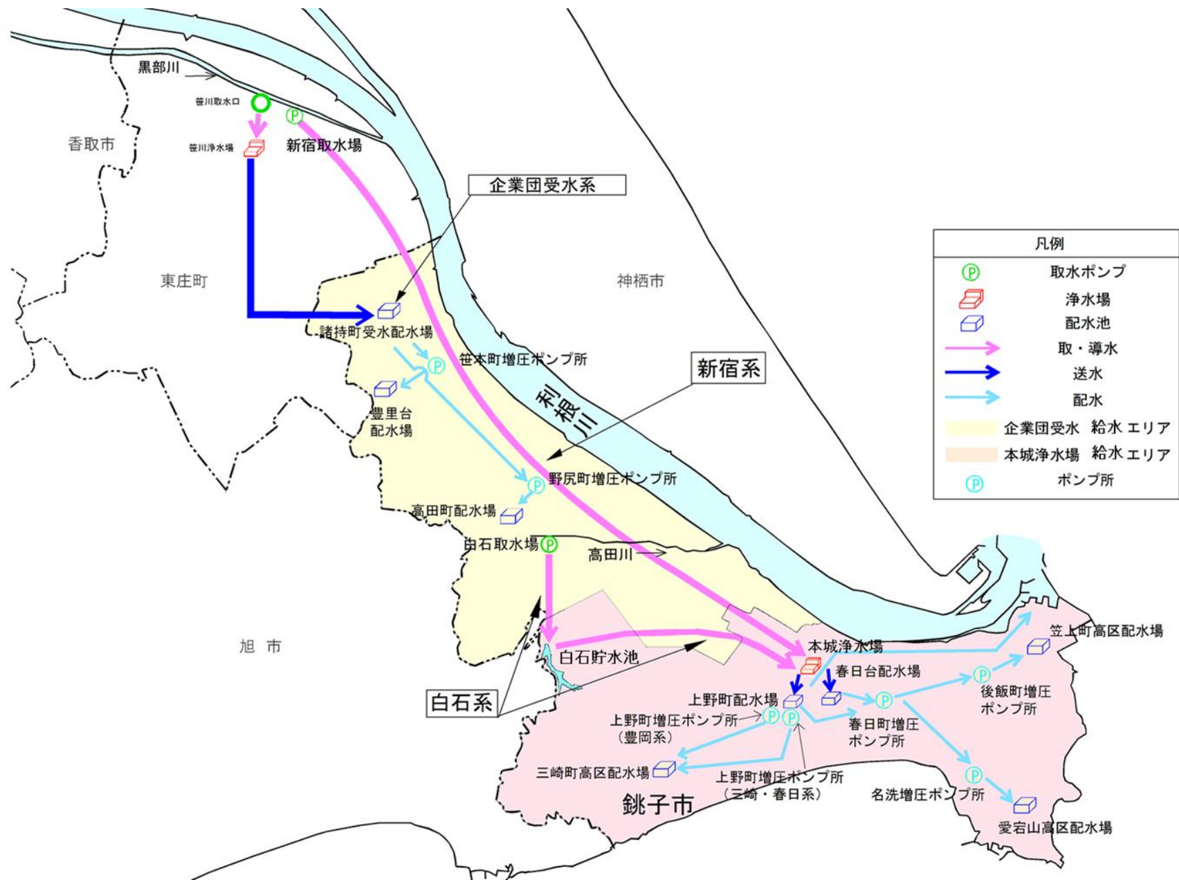
図1 銚子市水道局給水区域
